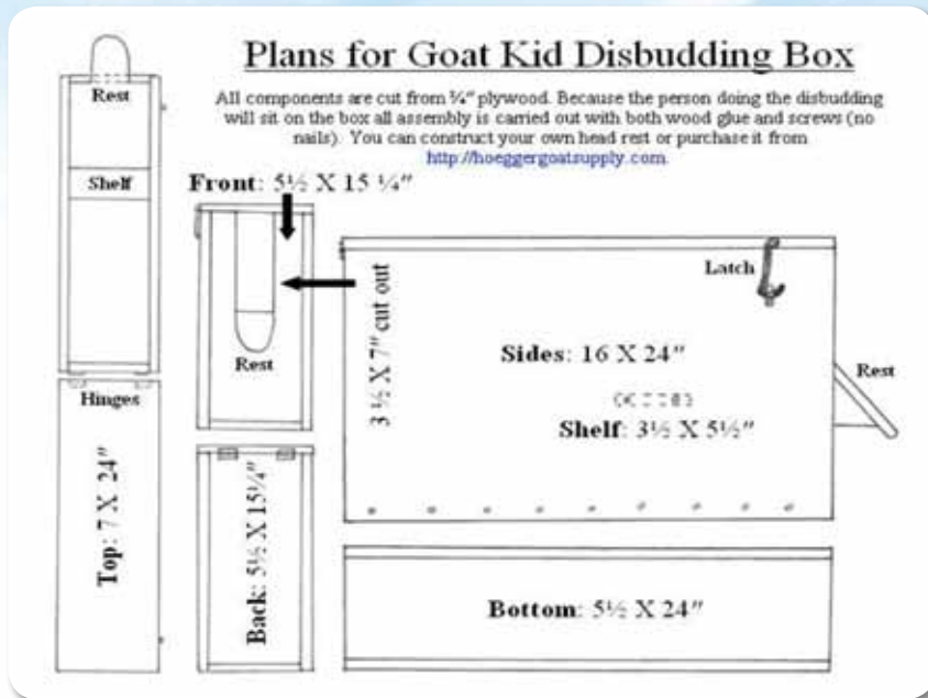
圖四、仔羊去角之保定箱之設計格式。
